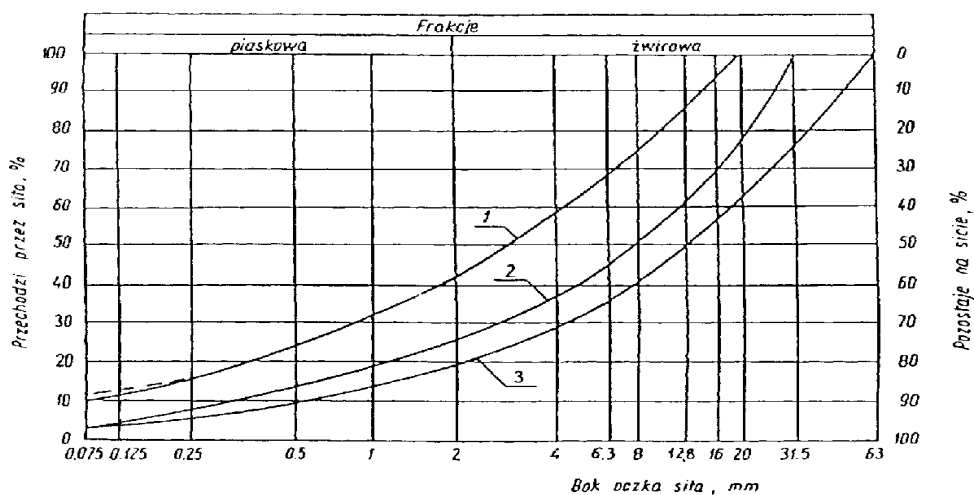
Rysunek 1. Pole dobrego uziarnienia kruszywa przeznaczonych na podbudowy
