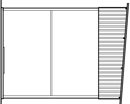
ELEWACJA ZACHODNIA
