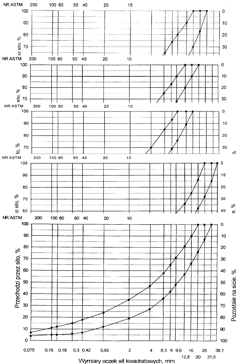
Rys. 3. Krzywe graniczne uziarnienia mieszanki mineralnej BA od 0 do 20 mm do podbudowy nawierzchni drogi o obciążeniu ruchem KR 1 lub KR 2
